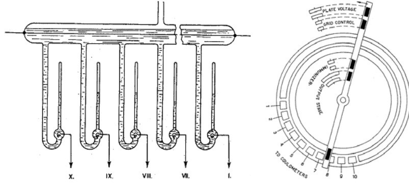
2.1. ábra. A coulométerek és a forgó rendszer [1]
