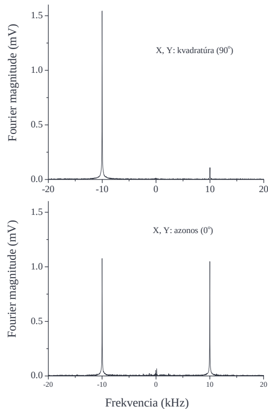
4.5. ábra. A spektrum analizátor működésének demonstrálása. A két méréshez a Siglent generátor két kimenetén egymás kvadrátúra párjait ill. azonos fázisban lévő jeleket állítottam be. Látható, hogy nem kvadrátúra jelek esetén a frekvencia előjele nem határozható meg.
