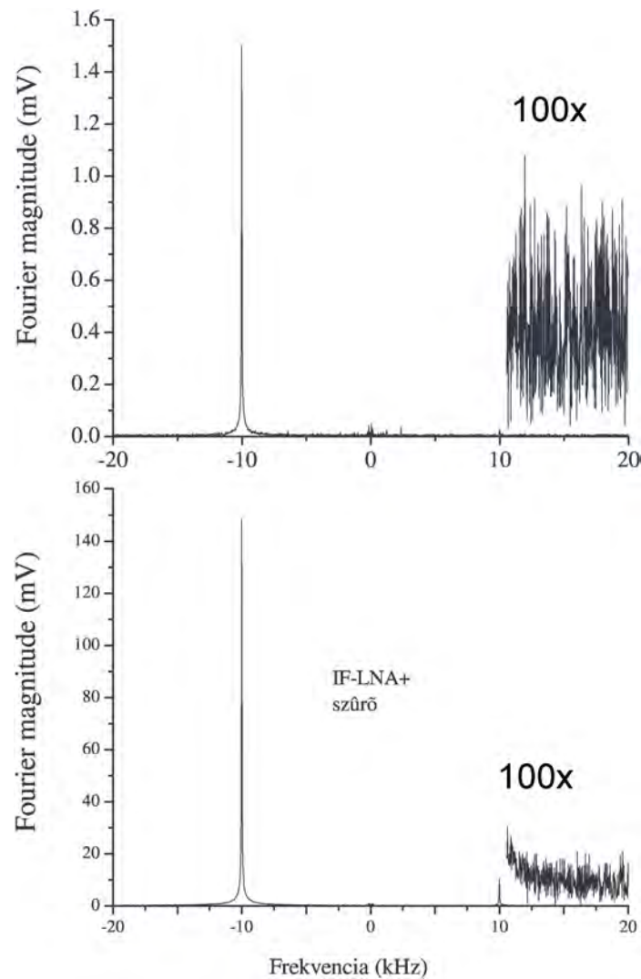
4.6. ábra. Az aluláteresztő szűrő hatása az oszcilloszkóppal digitalizált és Fourier transzformált jelre. A jel a Siglent generátor 4\text{ mV}_{pp} -es kvadrátúra jele volt (10 kHz-en), ami egyszer közvetben mértünk az oszcilloszkóppal, majd erősítve (100x) az IF-LNA-val és szűrve az aluláteresztő szűrővel. Látható, hogy a második esetben detektált jel jel-zaj aránya sokkal jobb.
