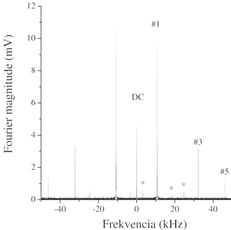
4.7. ábra. Az ultra alacsony zajú mikrohullámú spektrum analizátor érzékenységének karakterizálása -109.5 dBm 10.7 KHz-es négyzetöggel modulált jelre. A DC csúcsot és néhány zajkomponenst bejelöltünk (*), valamint a négyzetöggel fundamentális (#1) és 3-5. harmonikusait (#3 és #5).
