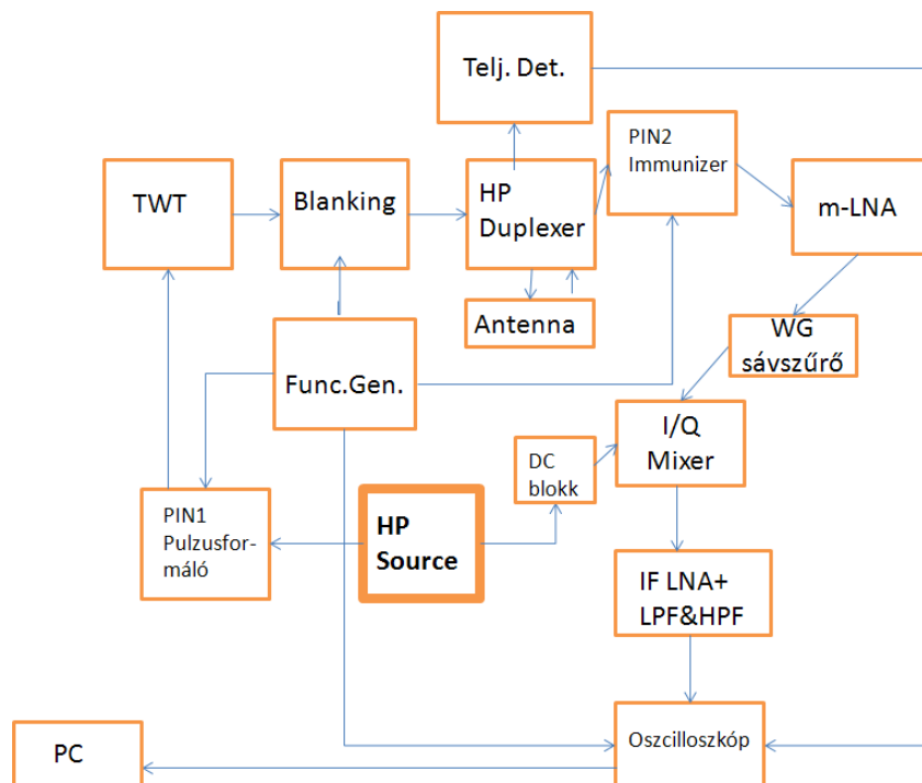
4.1. ábra. A Hold-radar kísérlethez megépített rendszer blokkdiagramja
