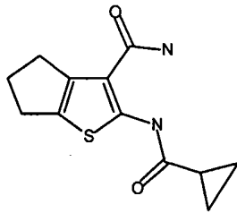
Compound D196
